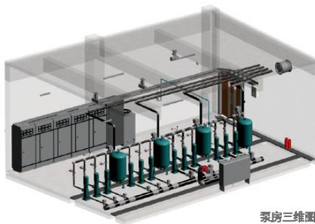
泵房三维图
