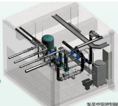
泵房空间控制图
