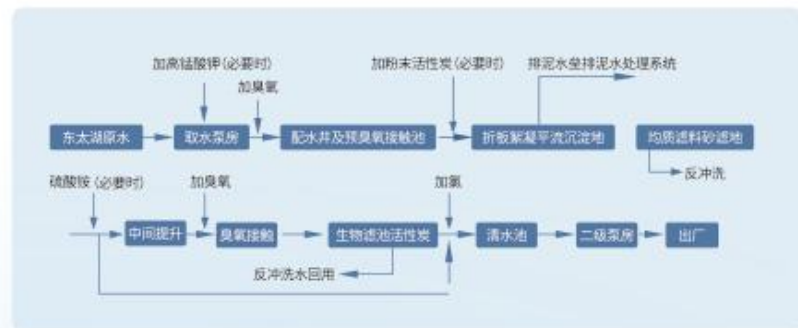
图1 苏南某水厂工艺流程
